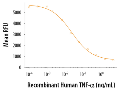
Recombinant Human TNF-α (#210-TA) の生物活性
