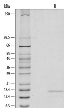
Recombinant Human TNF-α (#210-TA) のSDS-PAGE
